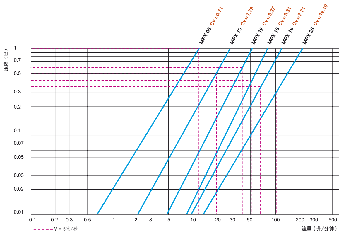
流量/压降曲线图
